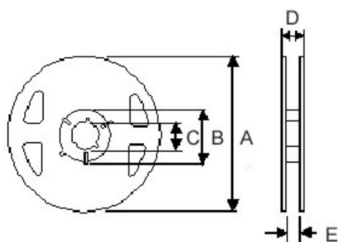
Reel Dimensions
