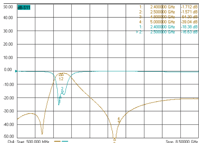
BPF1608T2450HA2
