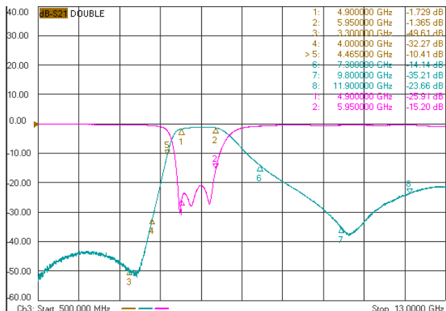
BPF2012T5500HA4
