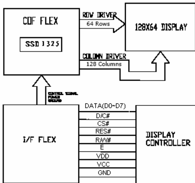
128X64 OLED Module
